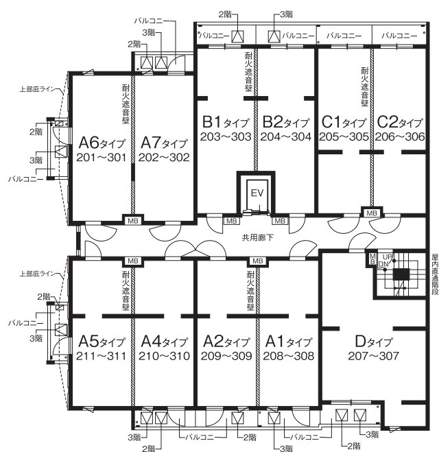
■2.3階平面図
