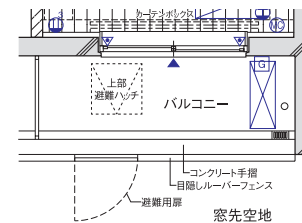
■1階部分図
