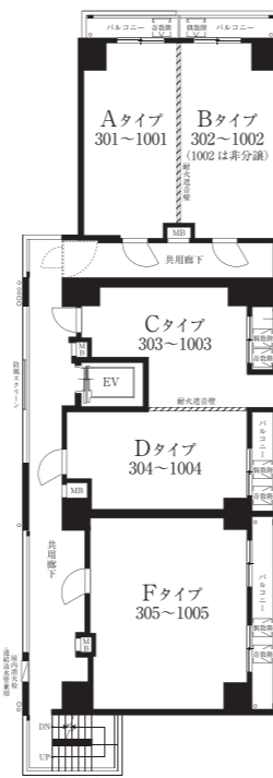
3～10階平面図
