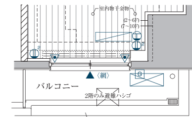
2・4・6・8・10階 バルコニー部分図
