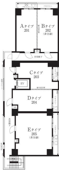
2階平面図
