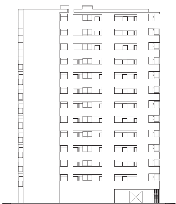
西側立面図
