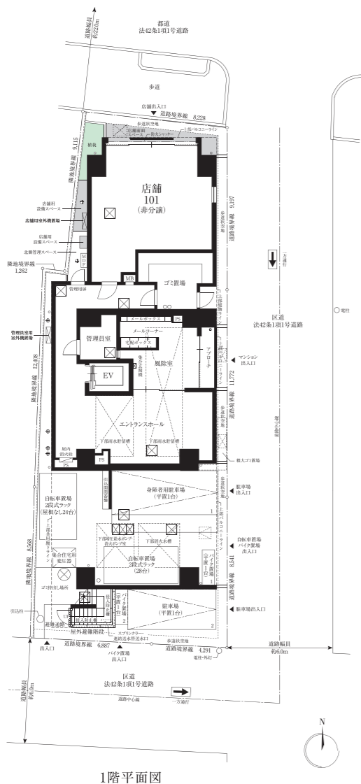
1階平面図
